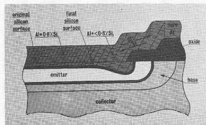
Afb. 6 Emitter protectie met behulp van polykristallijn silicium
