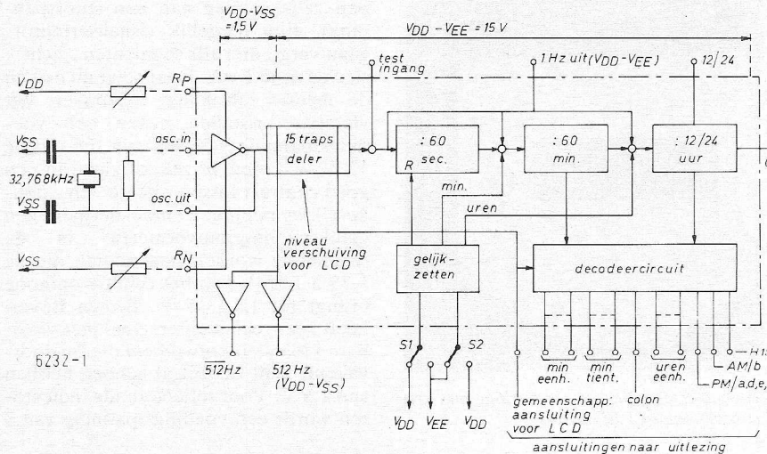
Fig. 1. Verschillende display configuraties en een voorbeeld van een geïntegreerd horloge circuit.
