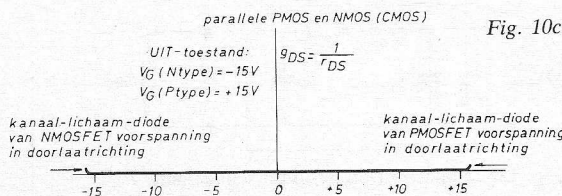
Fig. 10. Principeschakeling en karakteristieken van CMOS paren.
