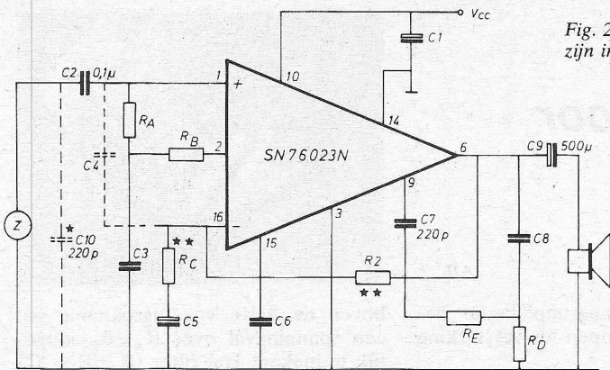
Fig. 3. Praktisch schema van een laagvermogen versterker, voorzien van gescheiden toonregeling voor hoog en laag.
