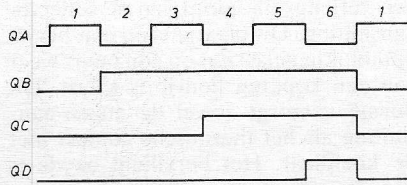
Fig. 1 Tijddiagram
