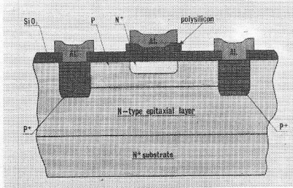
Afb. 4 Dwarsdoorsnede van een overlay microgolf transistor
