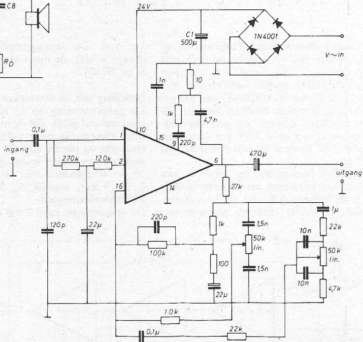
Fig. 3. Praktisch schema van een laagvermogen versterker, voorzien van gescheiden toonregeling voor hoog en laag.
