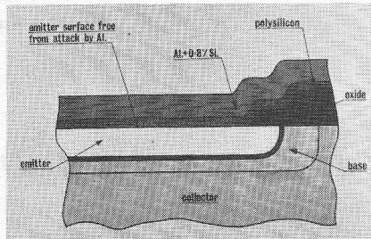
Afb. 5 Aantasting van de emitter door aluminium
