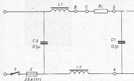
Fig. 2. Ontstoringfilter.
