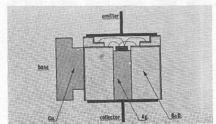
Afb. 7 Lintlijn-microgolf vermogenstransistoromhulling
