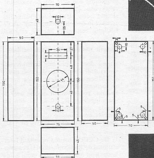
Fig. 3. Print lay-out.
