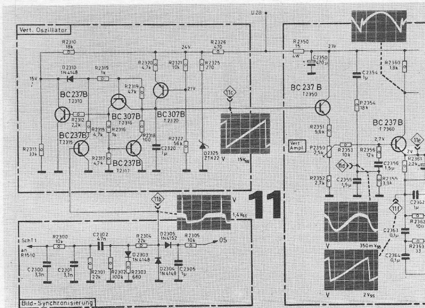
Fig. 2 Principeschema van de door Loewe ontwikkelde raster-afbuigschakeling met extreem groot vangbereik, waarbij de lineariteitscorrectieschakel achterwege kan worden gelaten.
