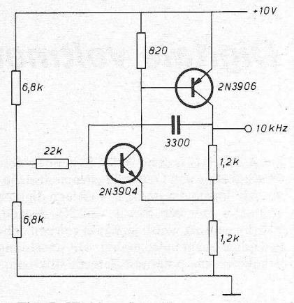
Fig. 7. Klokipulsosscillator.
