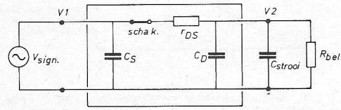
Fig. 13d. Gesloten schakelaar met strooicapaciteit.
