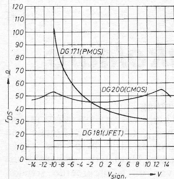
Fig. 11 r_{DS}/V_{sign} karakteristieken van drie FET schakelaars.
