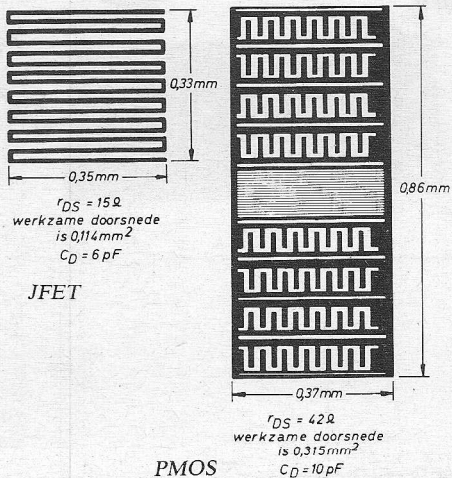
Fig. 14. Vergelijking van de werkzame doorsneden van PMOS en JFET schakelaars.
