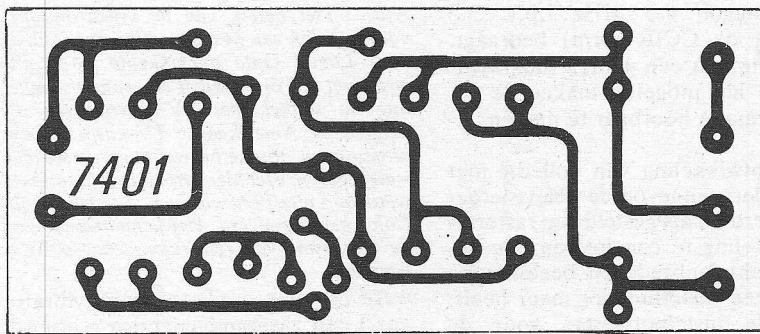
Fig. 3. Print lay-out.
