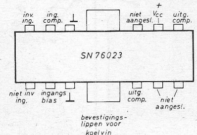
Fig. 1c. Aansluitgegevens van het toegepaste type.
