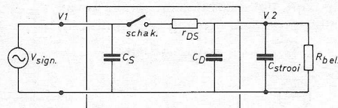
Fig. 13c. Capaciteit bij geopende schakelaar met strooicapaciteit.
