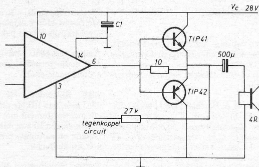
Fig. 5. Op deze manier is de schakeling uit te breiden voor grotere vermogensafgifte tot ca 15 W.
