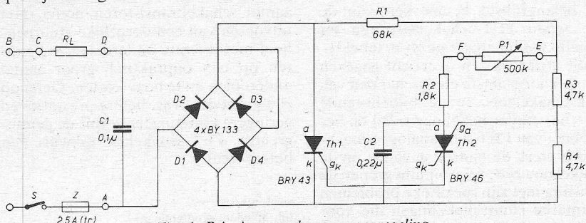
Fig. 1. Principe van de vermogenregeling.
