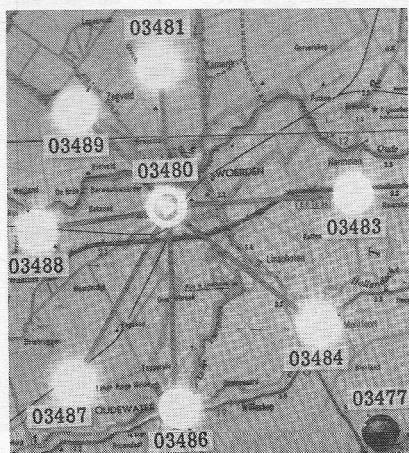
Afb. 3. Knooppuntcentrale Woerden met 7 eindcentrales
